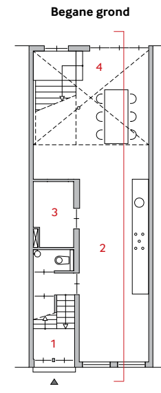
Begane grond
