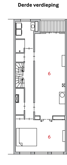
Derde verdieping
